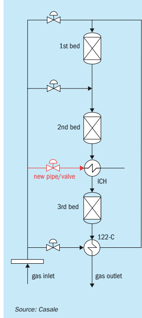
Fig. 9: New bottom feeding for ICH
